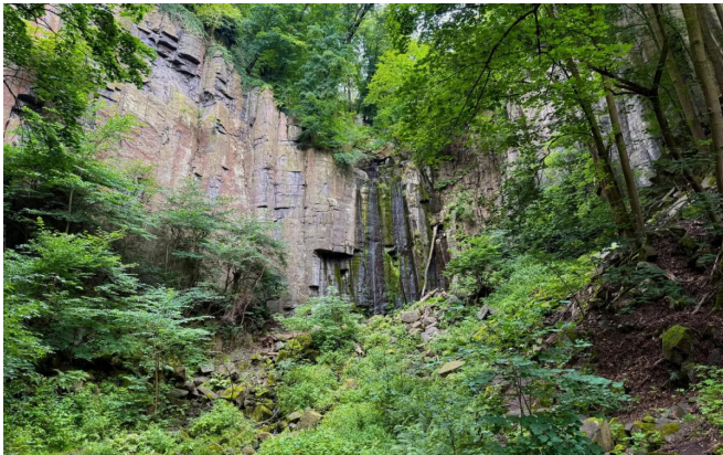
Imposanter Basaltaufschluss in Böhmen
