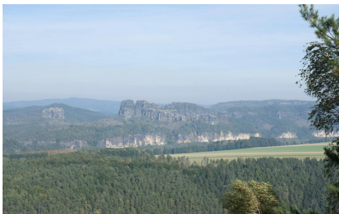
Blick auf Schrammsteinkette mit Falkenstein
